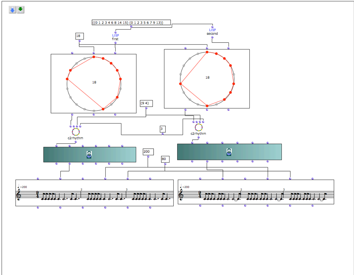
FIGURE 3.1 – Deux parties de \mathbb{Z}_{18} en \mathbb{Z}^3 -Relation, utilisées comme séquences rythmiques périodiques dans OpenMusic
